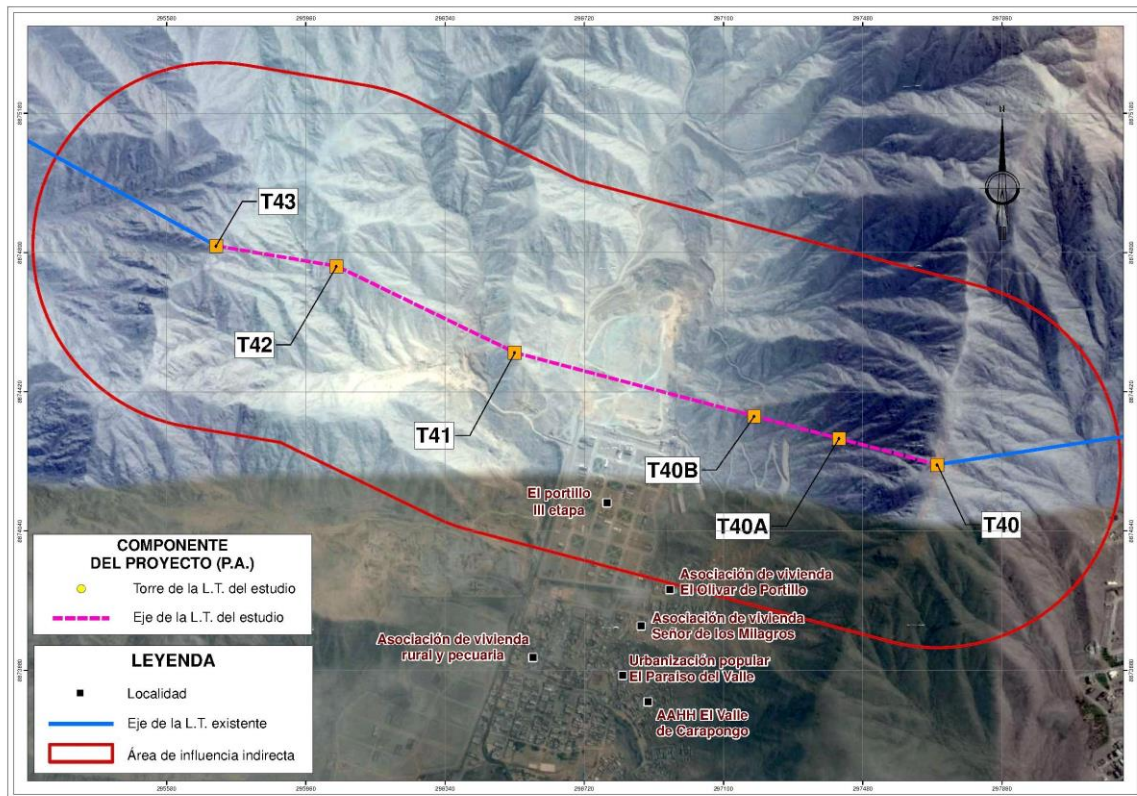
Imagen LOB 7-1: Trazo de la LT a desmontar
